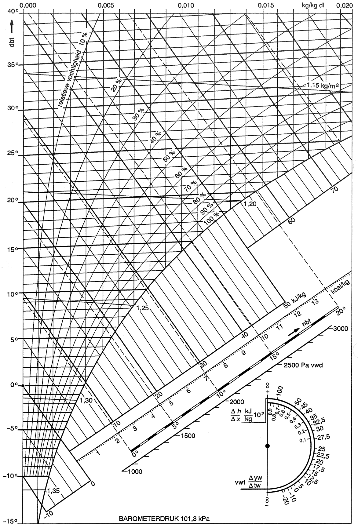
Figuur 16 Mollier-h/x-diagram bij 1,013 bar
